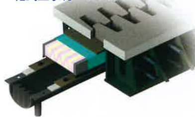
乾式止水材「プレスアドラー」
